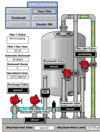
Figura : Visualização e Acompanhamento dos Sistemas Monitorados 2/2
