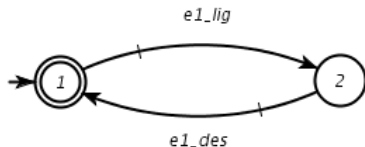
Modelo Esteira
