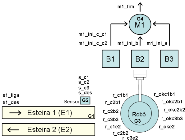
Figura : Layout da Planta (Problema)
