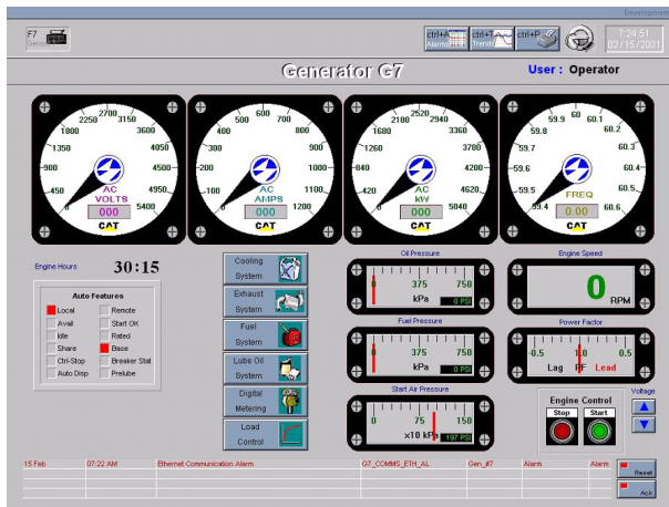
Figura : Visualização e Acompanhamento dos Sistemas Monitorados 1/2
