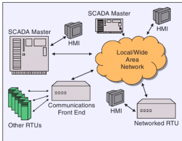
Figura : terceira geração da arquitetura SCADA
