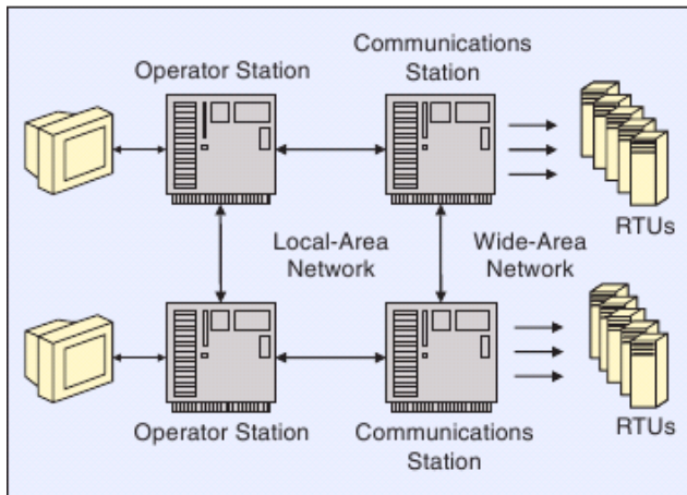
Figura : Segunda geração da arquitetura SCADA
